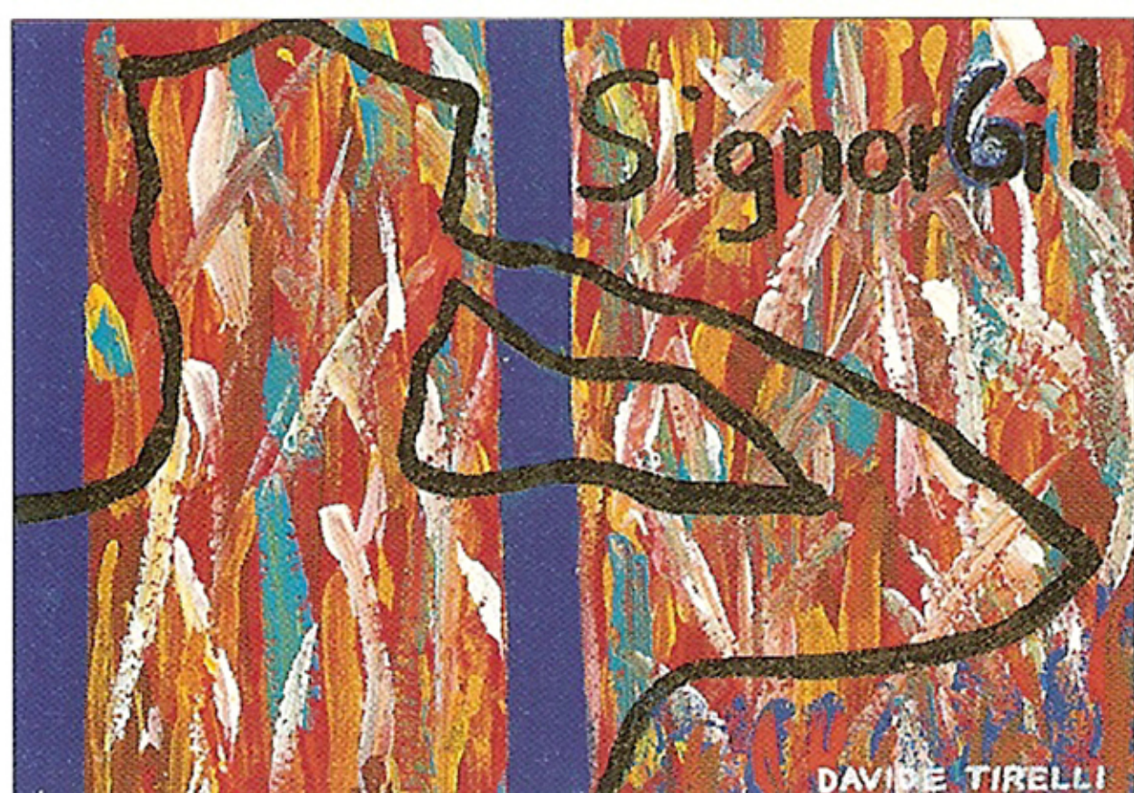
Davide Tirelli, Signor Gi!
